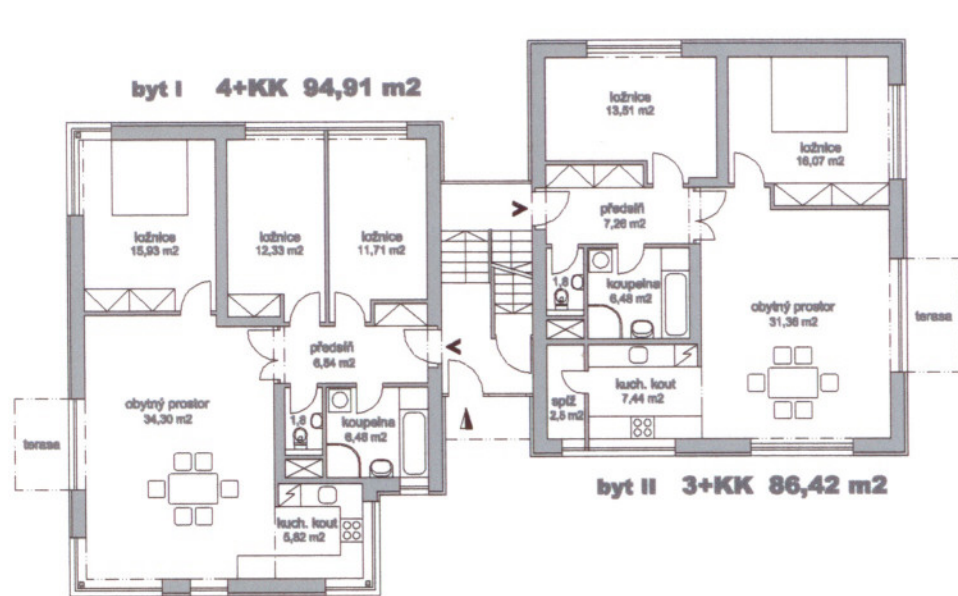
půdorys přízemí
