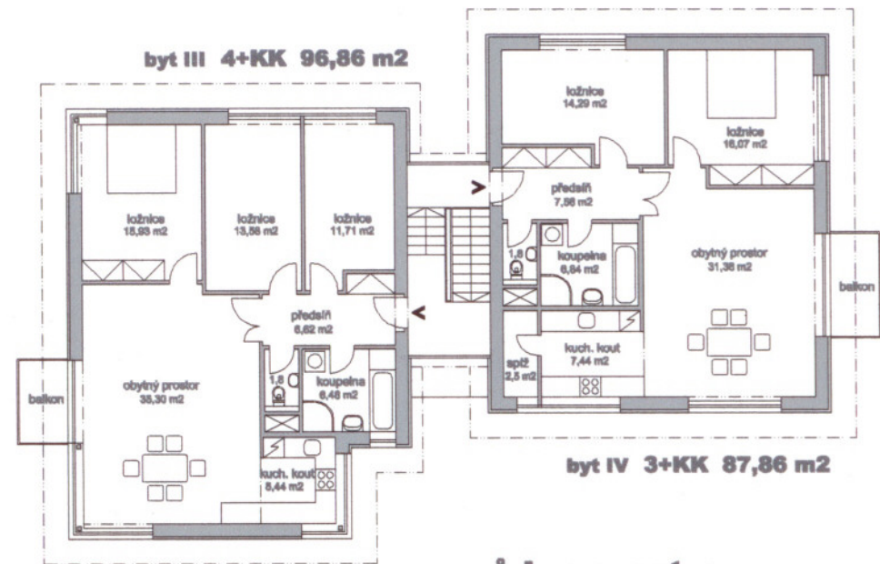
půdorys patra
