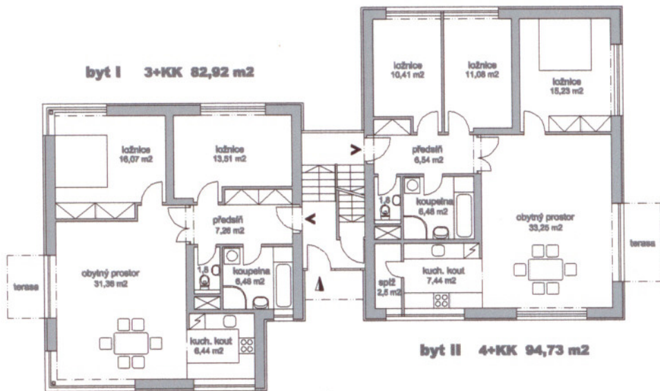
půdorys přízemí
